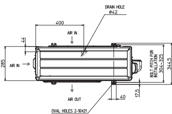
Inwerterowe urządzenia zewnętrzne SUZ, chłodzenie / grzanie, SUZ-M50VA
