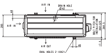
Inwerterowe urządzenia zewnętrzne SUZ, chłodzenie / grzanie, SUZ-M25/35VA
