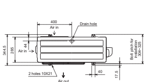
Inwerterowe urządzenia zewnętrzne MUFZ, chłodzenie / grzanie, MUFZ-KJ25 / 35VEHZ
