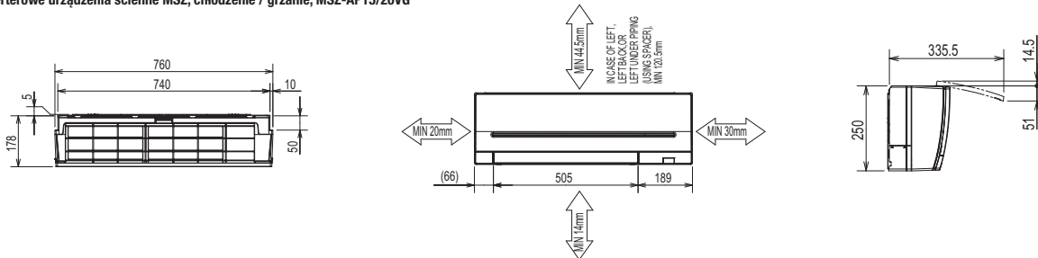
Inwerterowe urządzenia ściennie MSZ, chłodzenie / grzanie, MSZ-AP15/20VG
