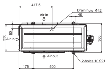
Inwerterowe urządzenia zewnętrzne SUZ, chłodzenie / grzanie, SUZ-M60/71VA
