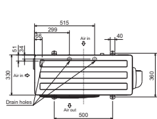
Inwerterowe urządzenia zewnętrzne MUFZ, chłodzenie / grzanie, MUFZ-KJ50VEHZ
