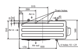
Inwerterowe urządzenia zewnętrzne MUZ, chłodzenie / grzanie, MUZ-EF50VG
