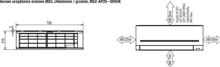
Inwerterowe urządzenia ściennie MSZ, chłodzenie / grzanie, MSZ-AP25-50VGK
